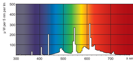
Farba svetla TL-D de Luxe /930
