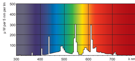
Farba svetla TL-D de Luxe /940
