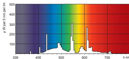
Farba svetla TL-D de Luxe /950
