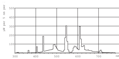
Farba svetla TL-D de Luxe /940
