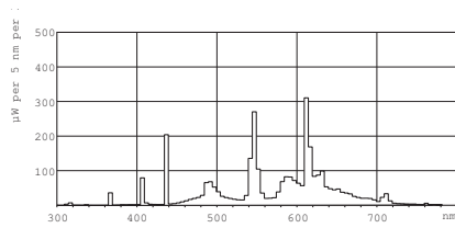
Farba svetla TL-D de Luxe /930
