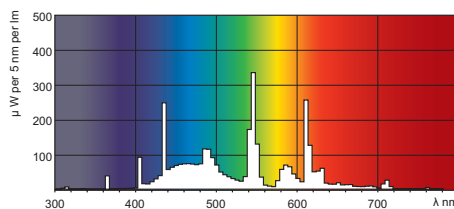
Farba svetla TL-D de Luxe /965
