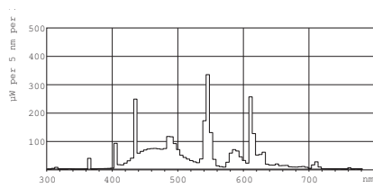
Farba svetla TL-D de Luxe /965
